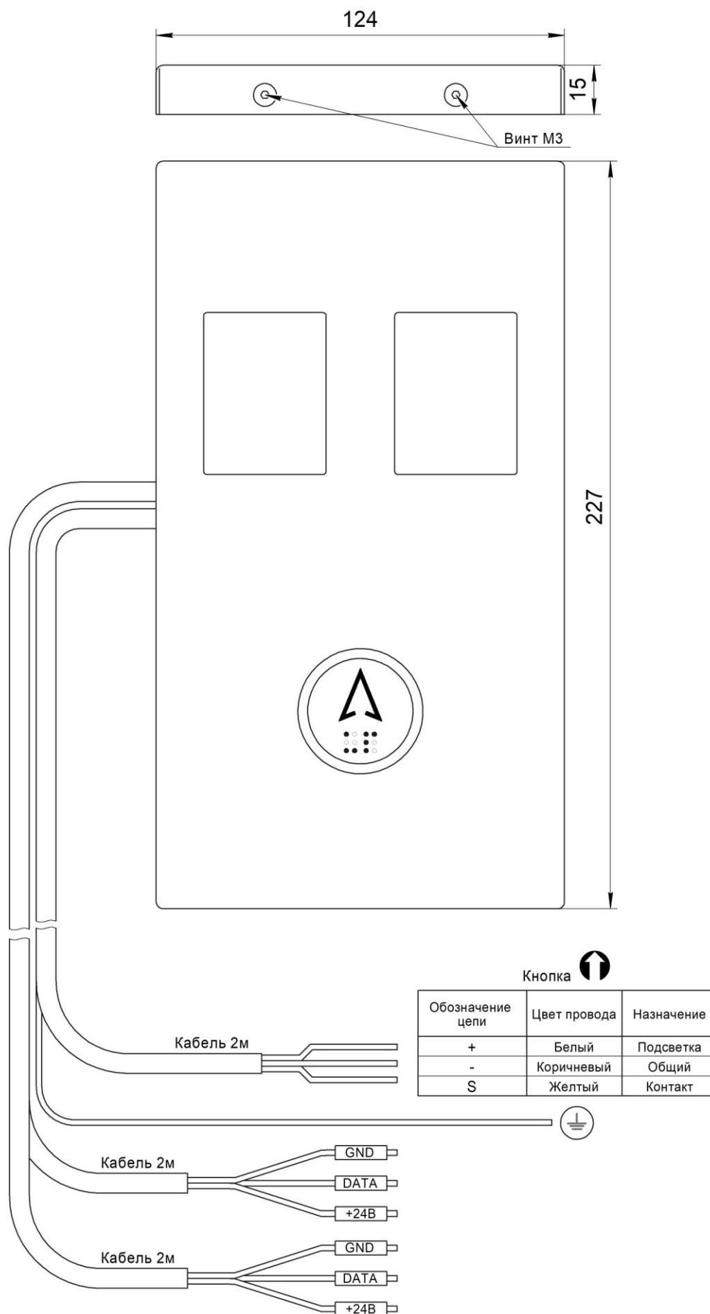
Рис.1 Внешний вид, габаритные и установочные размеры Вызывного поста КВАДРО НШЕК.468381.068
